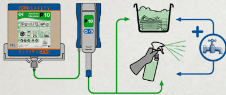
Sistemas de dilución sin punto de agua
